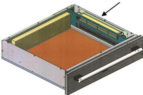
Gebälseeinheit mit Heizelement
